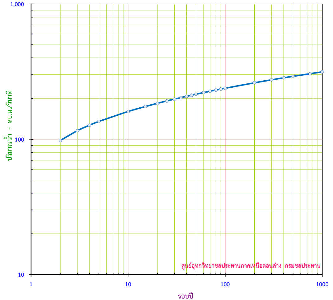
กราฟแสดง ปริมาณน้ำสูงสุดรายปี ขนาดรอบปีต่างๆ สถานี N.59 บ.นาโพธิ์นาจาน อ.นครไทย จ.พิษณุโลก
